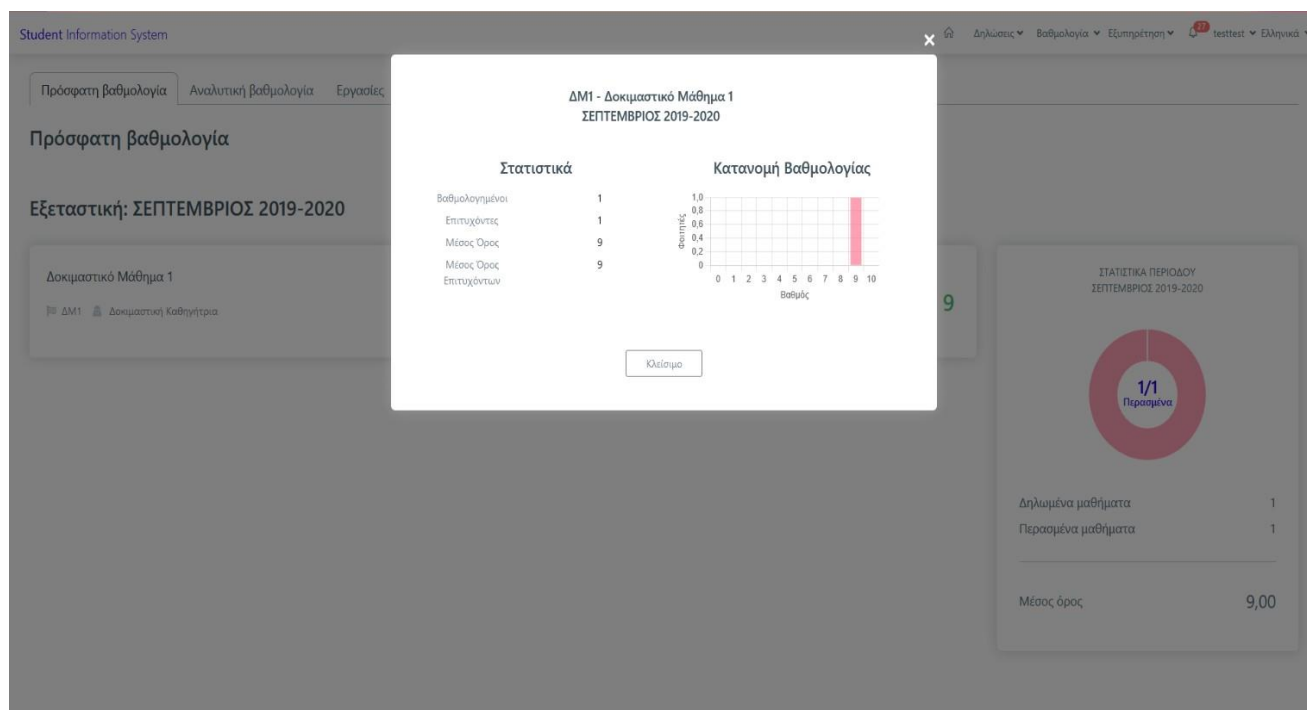
Εικ. 8.2: Στατιστικά
